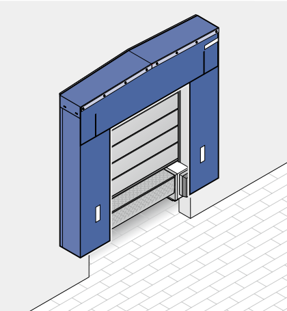
DDF 标准宽度: 3300/3400 mm 标准高度: 3500 mm
