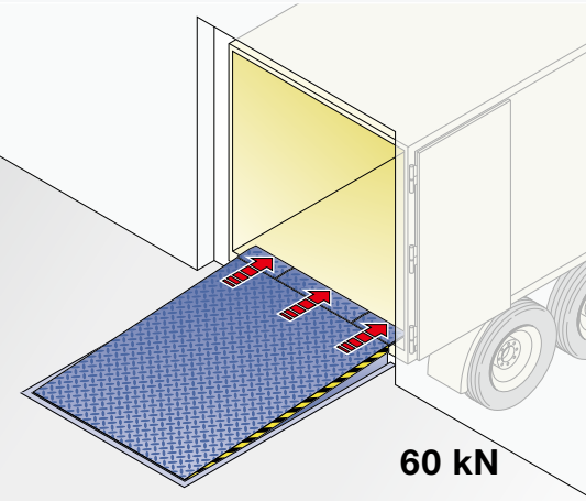
三段伸缩式装卸平台 HTLV 3
