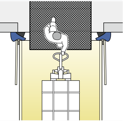
采用垫枕式门封，车厢与打开的门之间的缝隙也可以很好的密封。
