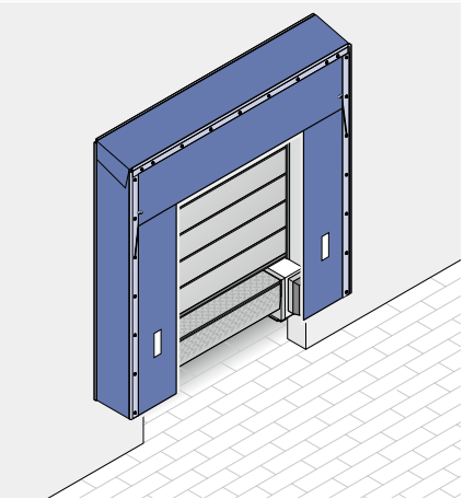
DSL 配连杆式支臂 DSL-H 配伸缩连杆式支臂 DSS 配剪式支臂 标准宽度: 3350 / 3500 mm 标准高度: 3500 / 3750 mm, 可以选择 4500 mm 高落地式 或缩进式
