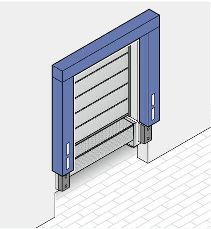
DFH 带有固定尺寸侧部垫枕与顶部垫枕的门封 标准尺寸： 2800 × 2500 mm (W × H)
