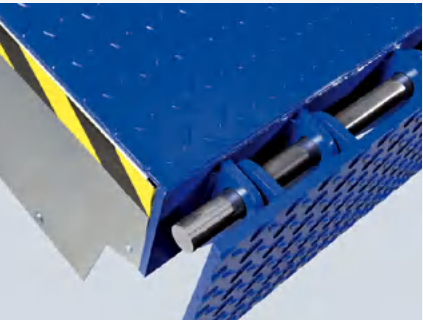
耐用的折板式唇板 开放式的唇板铰链设计，容易清理，防止木屑、石块等杂物在此处堆积。
