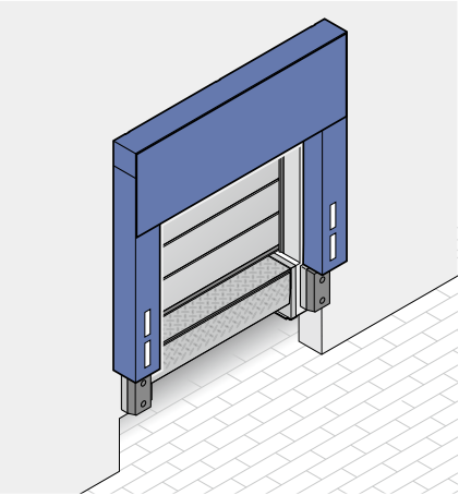
DFC 带有固定尺寸侧部垫枕的门封。 顶部垫枕配有附加帘板 标准尺寸： 2800 × 3000 mm (W × H)
