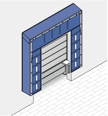
DTL 配连杆式支臂 DTS 配剪式支臂 标准宽度: 3350 / 3500 mm 标准高度: 3500 / 3750 mm, 可以选择落地式: 4500 mm 高
