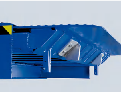
坚固的伸缩式唇板 伸缩唇板框架经过整体加强，非常坚固稳定。唇板由整块厚度为 12/14 mm 的防滑花纹板制成。
